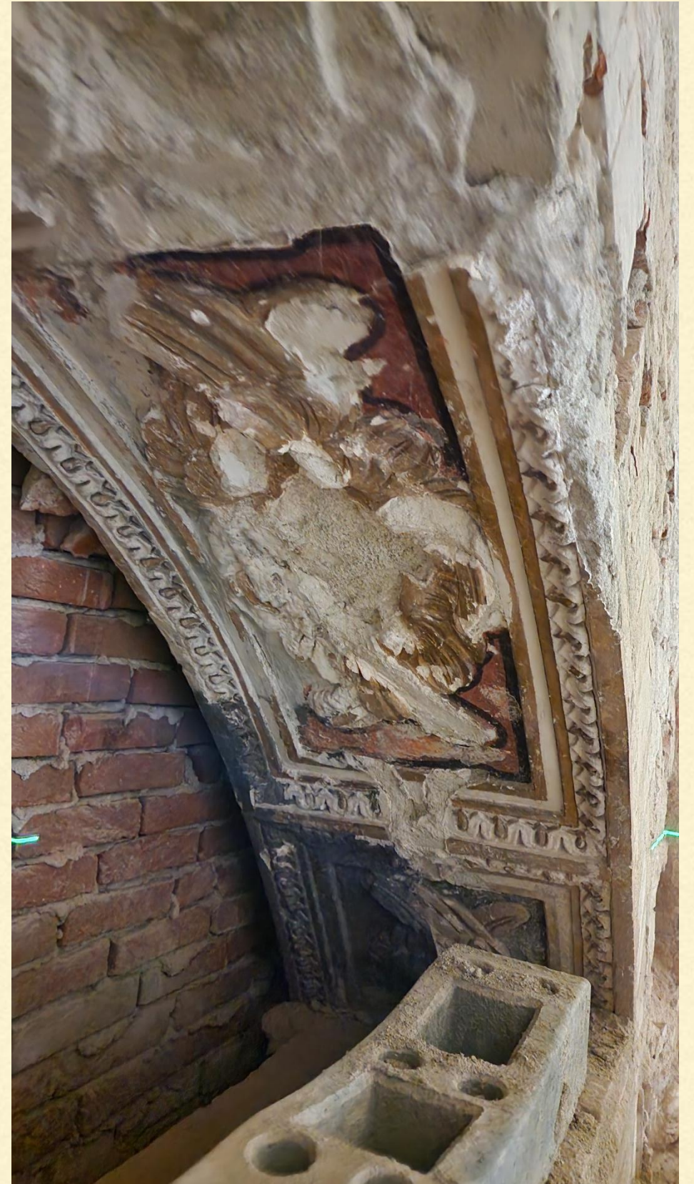
Restauro arco fase ottocentesca →
