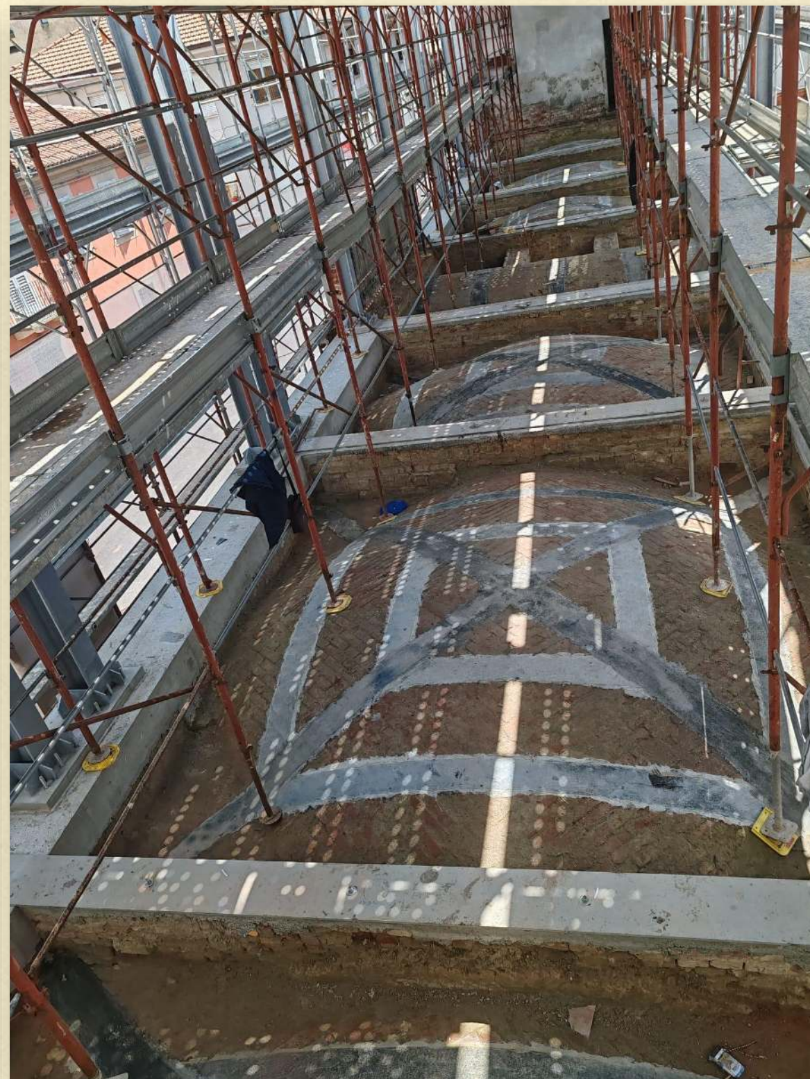
Consolidamento in fibra di carbonio - volte
